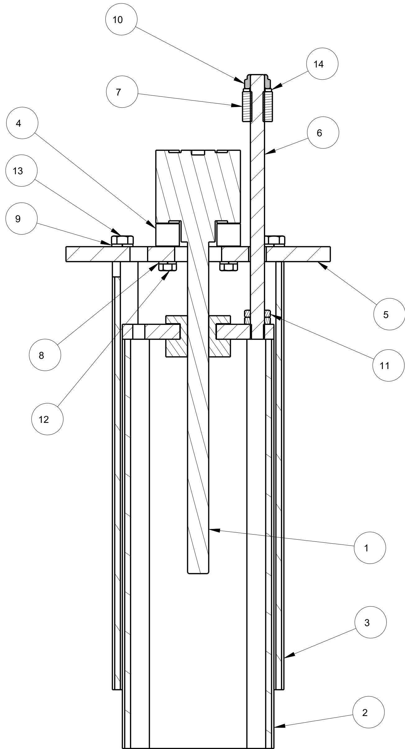
SECTION A-A
